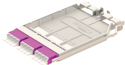
UHDM-PATCH-3xLCQDVIO-OM4
